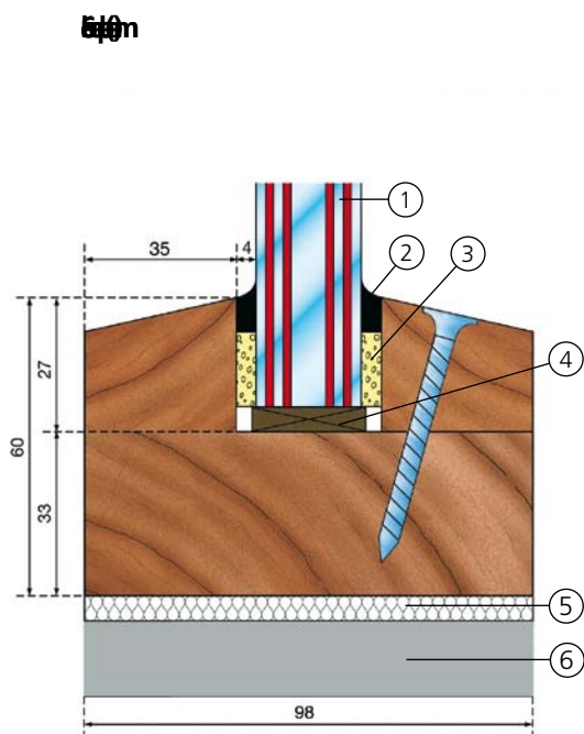
P.V. 94-A-133 Châssis bois dur
