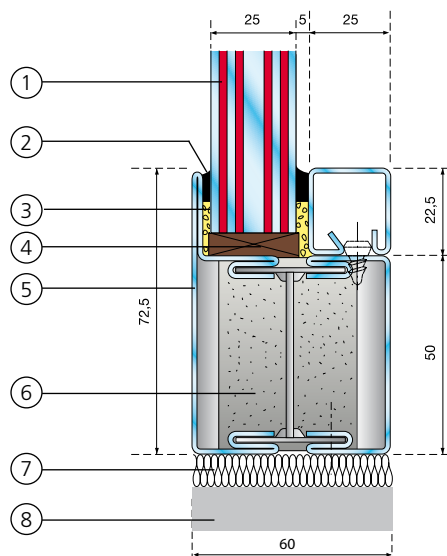
P.V. 01-A-049 Profil Jansen Janisol 3
